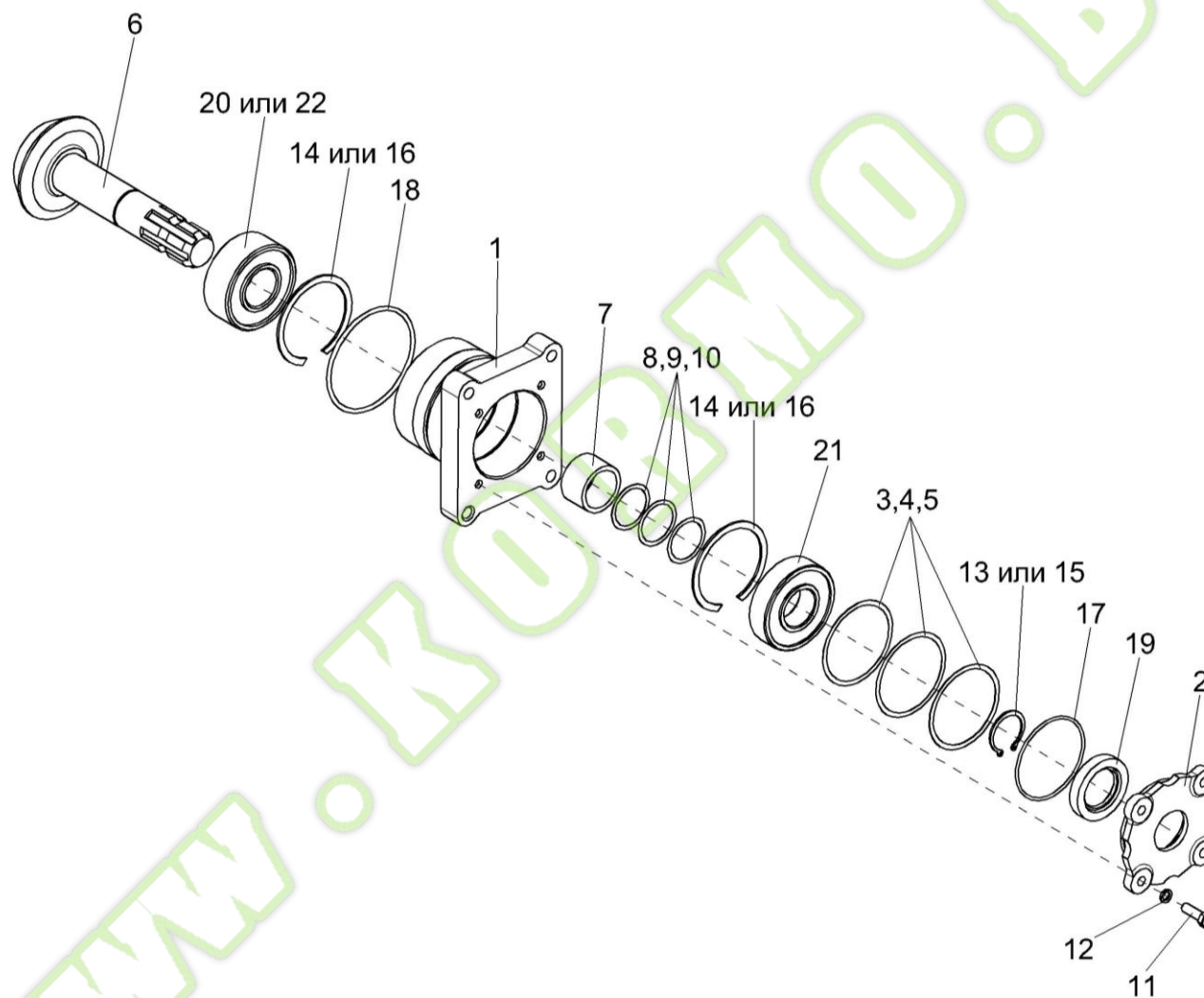
Рисунок 15 – Стакан ЖГР-1-0203010
