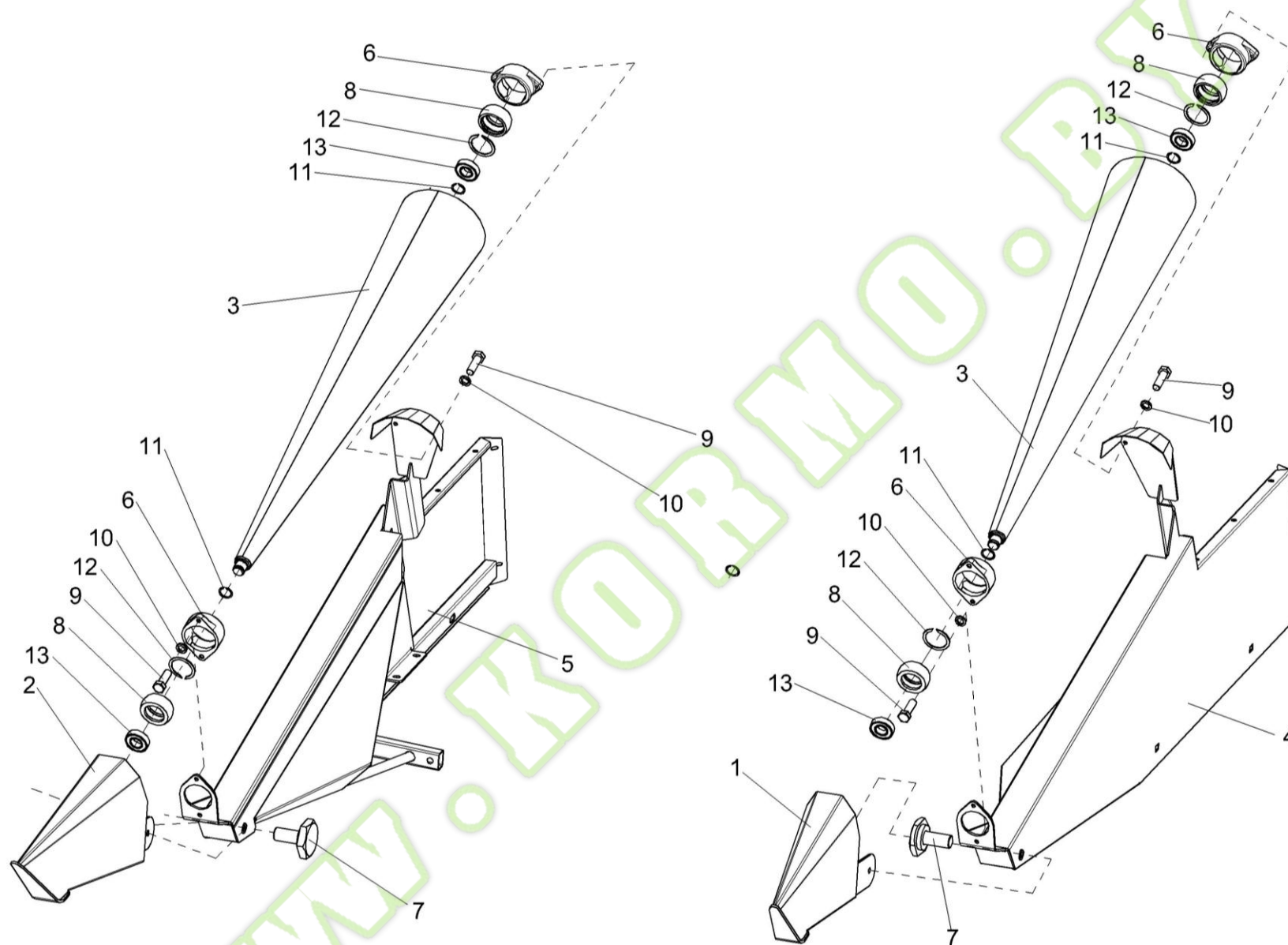
Рисунок 22 – Боковины ЖГР-3-0208000 и ЖГР-3-0208000-01
